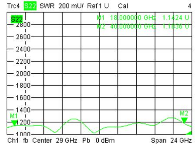
4.输出驻波比 Output VSWR
