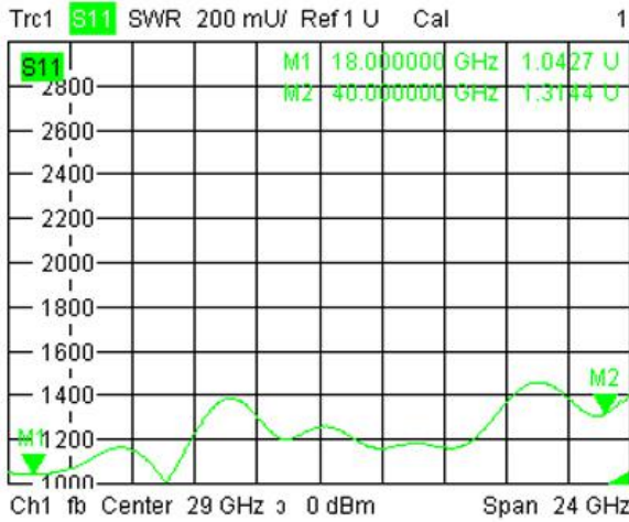
1.输入驻波比 Input VSWR
